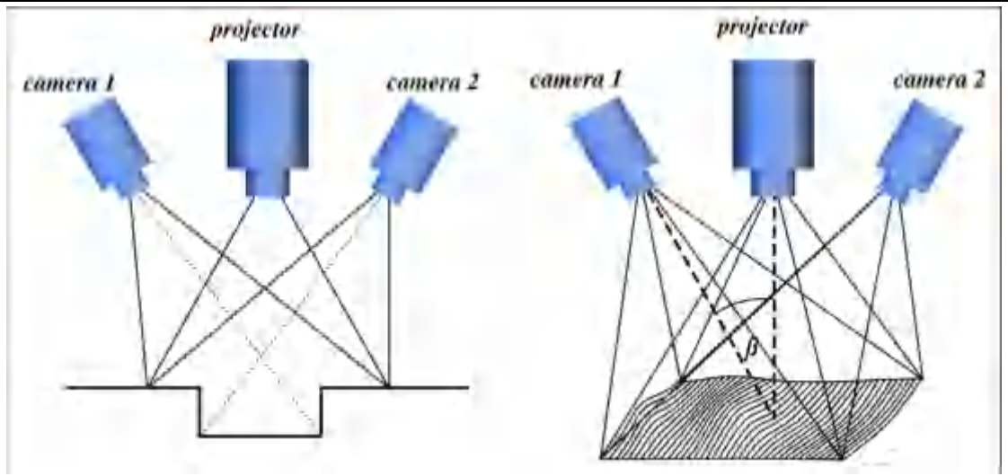
图表 5. 结构光三维扫描仪
